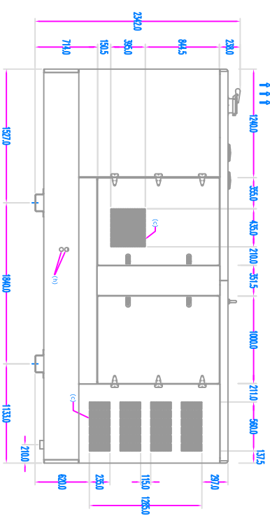
VISTA POSTERIOR REAR VIEW
